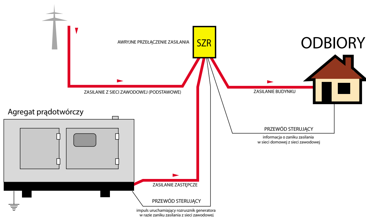
Schemat instalacji zewnętrznej dla agregatu w wersji obudowanej
